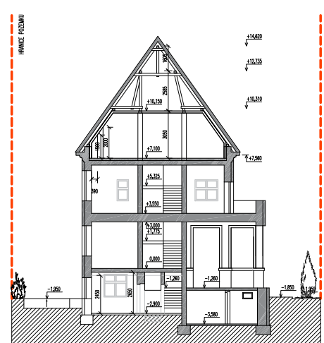
ŘEZ B - B
