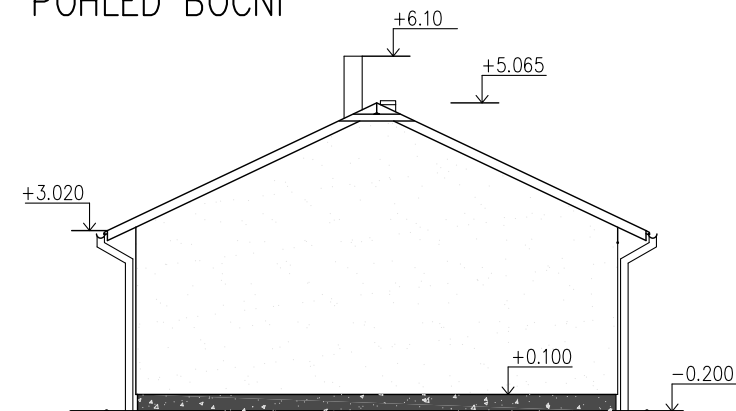
POHLED BOČNÍ
