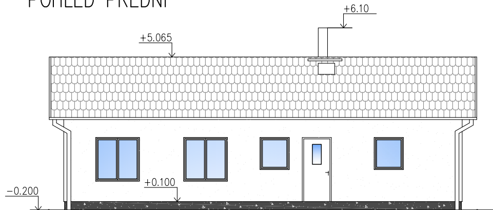
POHLED PŘEDNÍ
