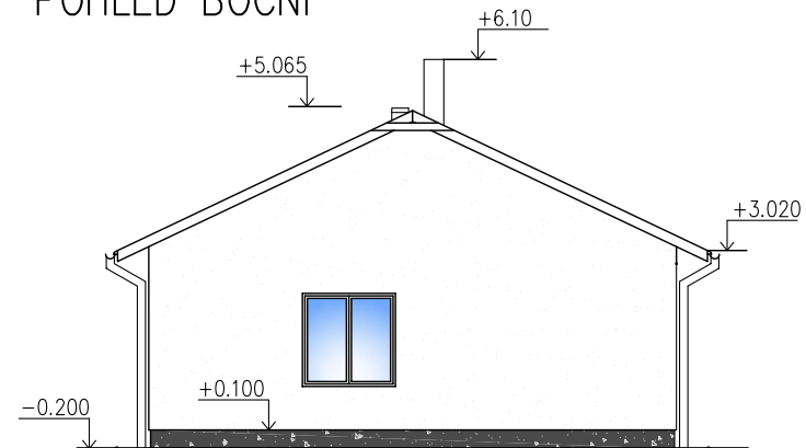
POHLED BOČNÍ
