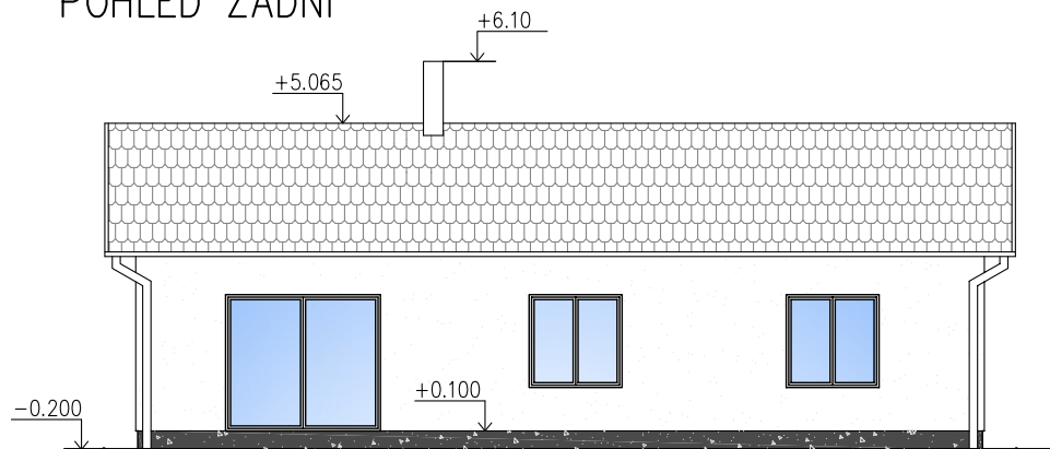
POHLED ZADNÍ
